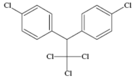
DDT
