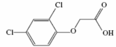
2,4-D
